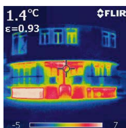
Analyse thermographique du bâtiment administratif
